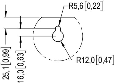
DETALHE/ DETAIL A ESCALA/SCALE 1 : 5
