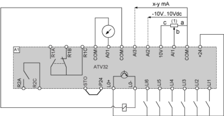
(1) Potenciômetro de referência SZ1RV1202 (2,2 kΩ) ou similar (10 kΩ máximo)
