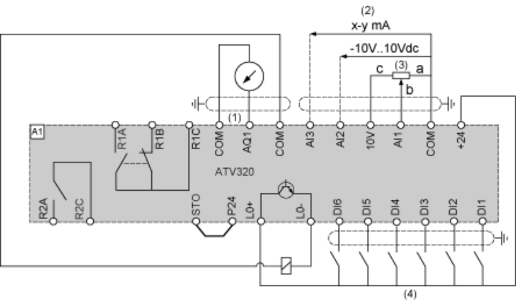
Diagrama de conexão do controle no modo Fonte
