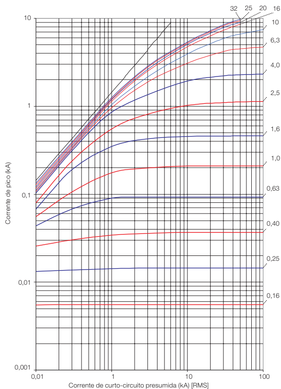
Curva de Limitação de Corrente em Curto-Circuito em 400/415 V - MPW25/40
